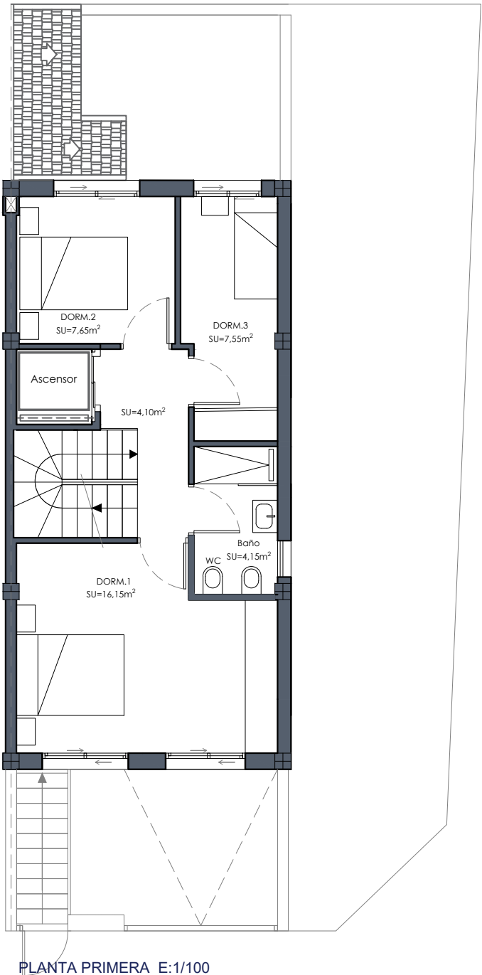
PLANTA PRIMERA E:1/100
