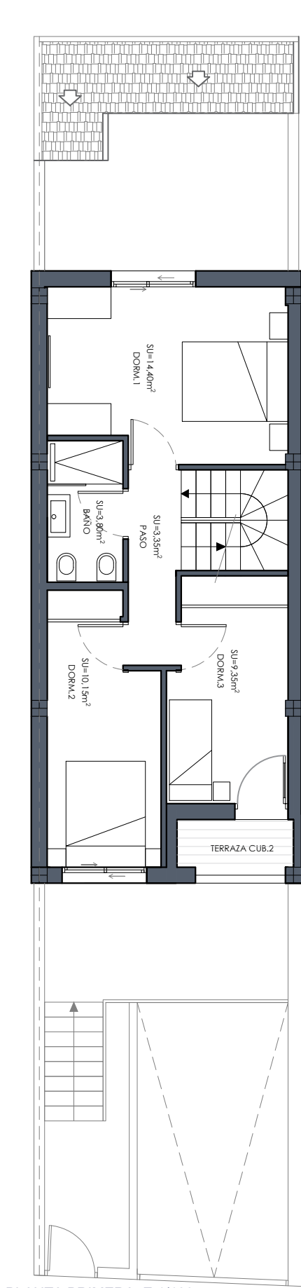
PLANTA PRIMERA E:1/100
