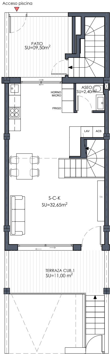
PLANTA BAJA E:1/100
