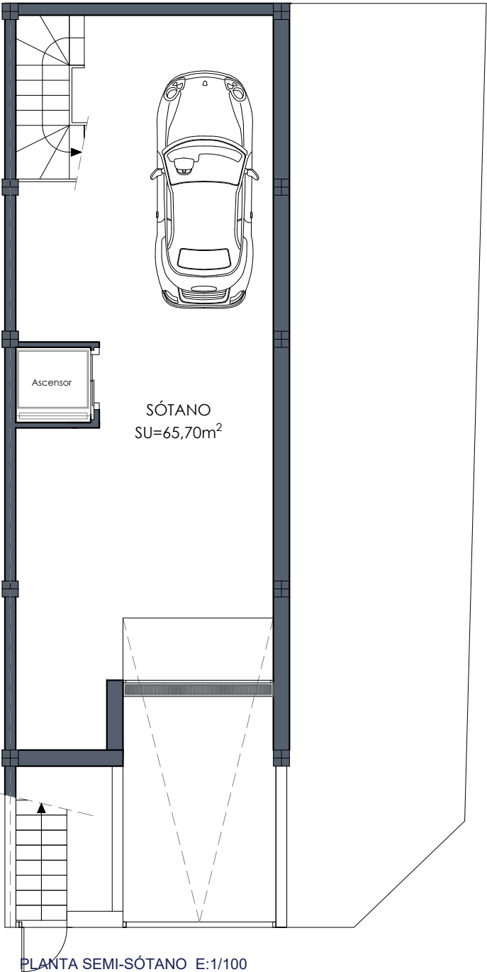
PLANTA SEMI-SÓTANO E:1/100
