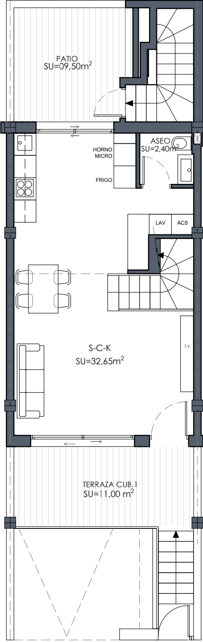
PLANTA BAJA E:1/100
