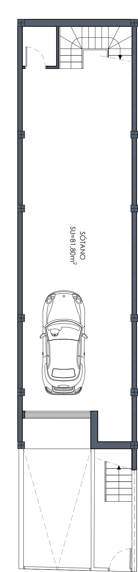
PLANTA SEMI-SÓTANO E:1/100
