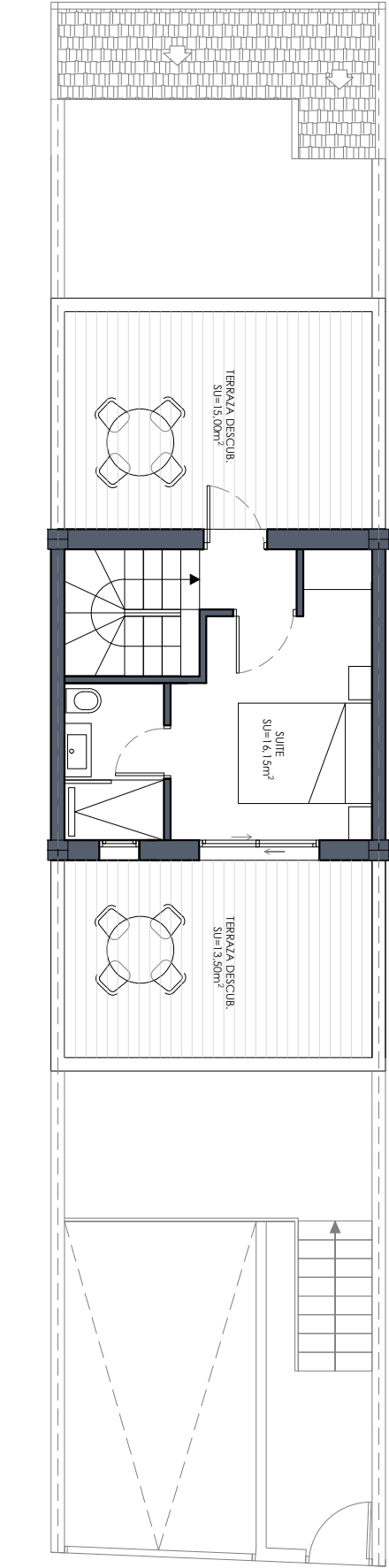
PLANTA ÁTICO E:1/100
