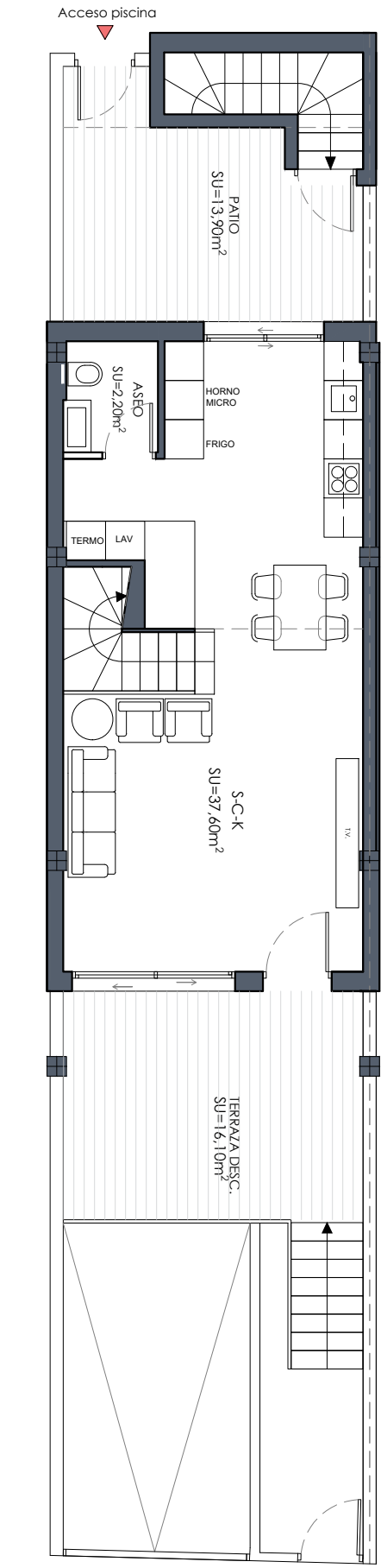
PLANTA BAJA E:1/100
