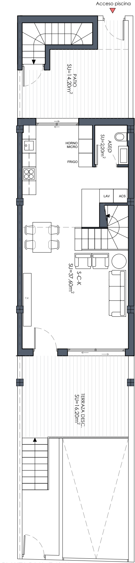
PLANTA BAJA E:1/100
